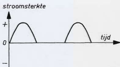
Fig. 11. De daaruit verkregen gelijkstroom
