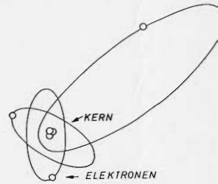
Fig. 3. Een atoom
