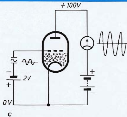
Fig. 14. Versterking van elektrische trillingen
