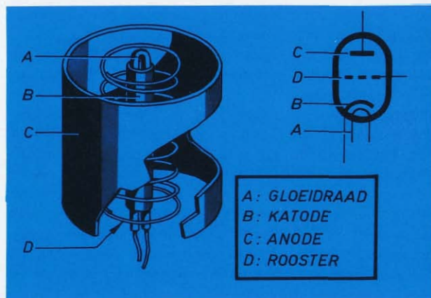
Fig. 13. De triode
